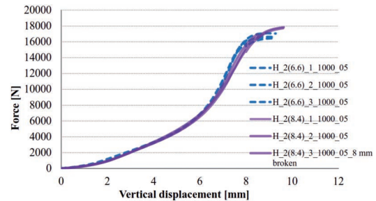
Fig. 11. Force vs. vertical displacement of laminated specimens consisted of 6+6 mm or 8+4 mm HSG glass layers with height of 1000 mm 11. ábra Terhelő erő és függőleges elmozdulás összefüggése (6+6 mm, 8+4 mm) vastag hőkezelt, laminált üvegekből felépülő, 1000 mm magas névleges magasságú oszlopok esetén
